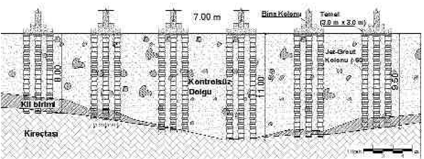
Şekil 1 : Sistem Enkesiti
